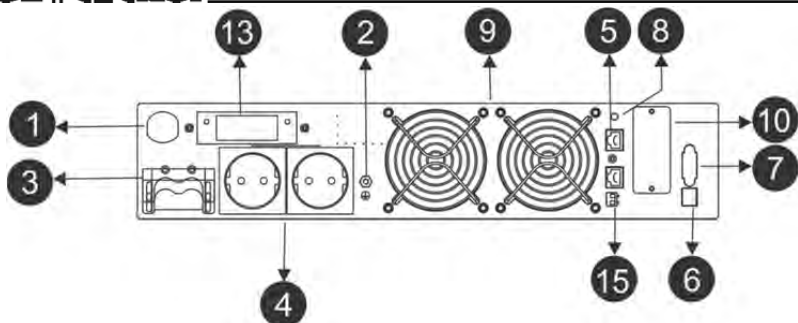
شکل ۳: نمای پنل پشت SDC1000,2000-PLUS
