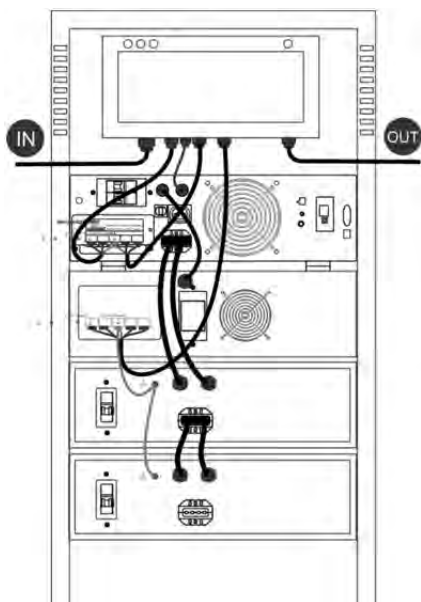
شکل ۱۵- د: یوپی اس SDC6000X-RT PLUS ، ترانسفورمر ایزوله و کابینت باتری و تابلوی بای پس
