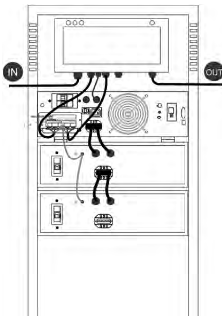
شکل ۱۵- ج: یوپی اس SDC6000X-RT PLUS ، ترانسفورمر ایزوله و دو کابینت باتری
