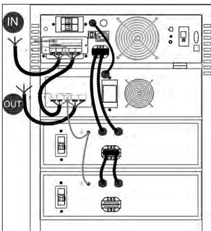
شکل ۱۵- ب: یوپی‌اس SDC6000X-RT PLUS ، ترانسفورمر ایزوله و دو کابینت باتری
