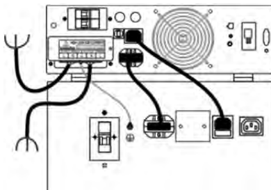
شکل ۱۰: SDC6000X-RT PLUS
