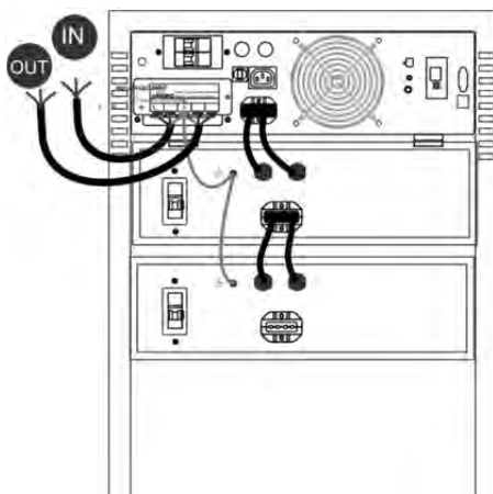
شکل ۱۵- الف: یوپی‌اس SDC6000X-RT PLUS با دو کابینت باتری
